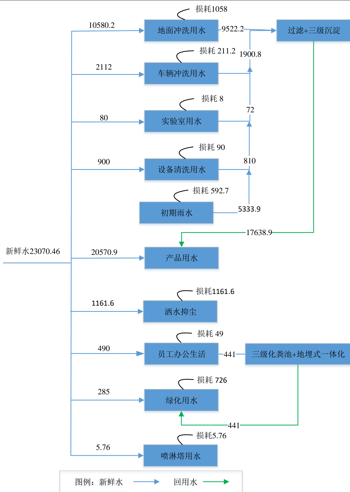
图2-1 扩建后，全厂水平衡图（单位：t/a）
