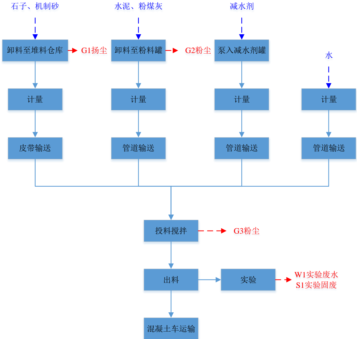
图 2-2 预拌混凝土生产工艺流程图
